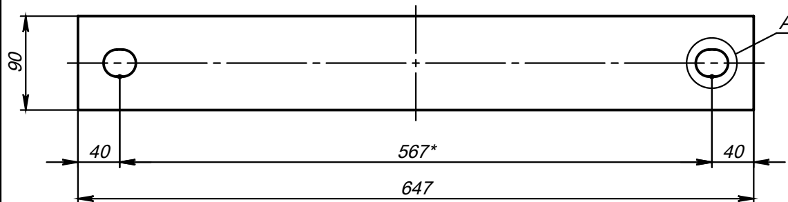
Поз.1 (Полухомут) развертка
