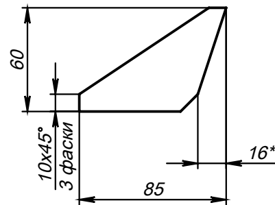
Поз.4 (Косынка) 1:3
