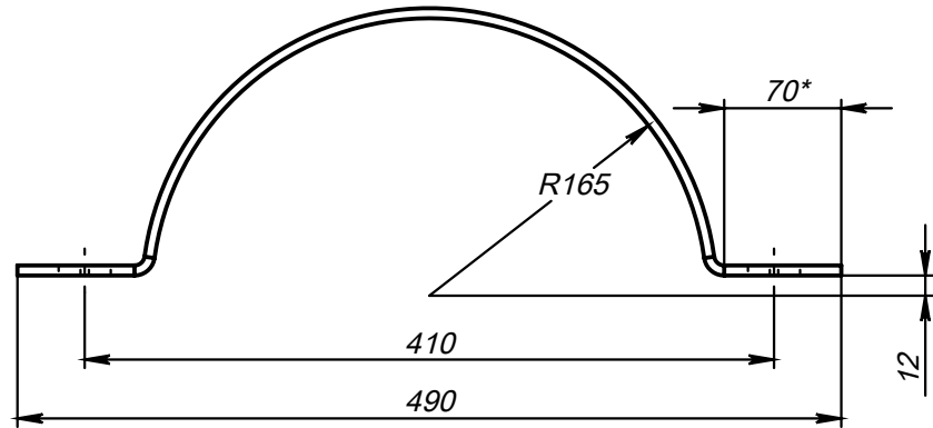
Поз.1 (Полухомут)
